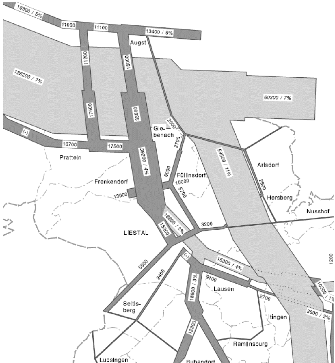
Abb. 8. Verkehrsbelastung des kantonalen Strassennetzes 2010
